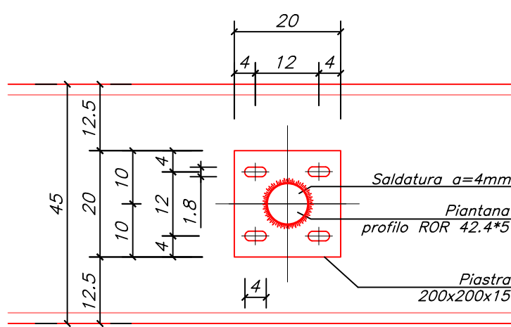
Dettaglio 3 (1:10)
