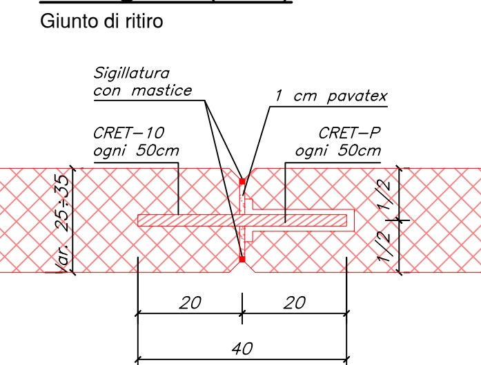
Dettaglio 2 (1:10)
