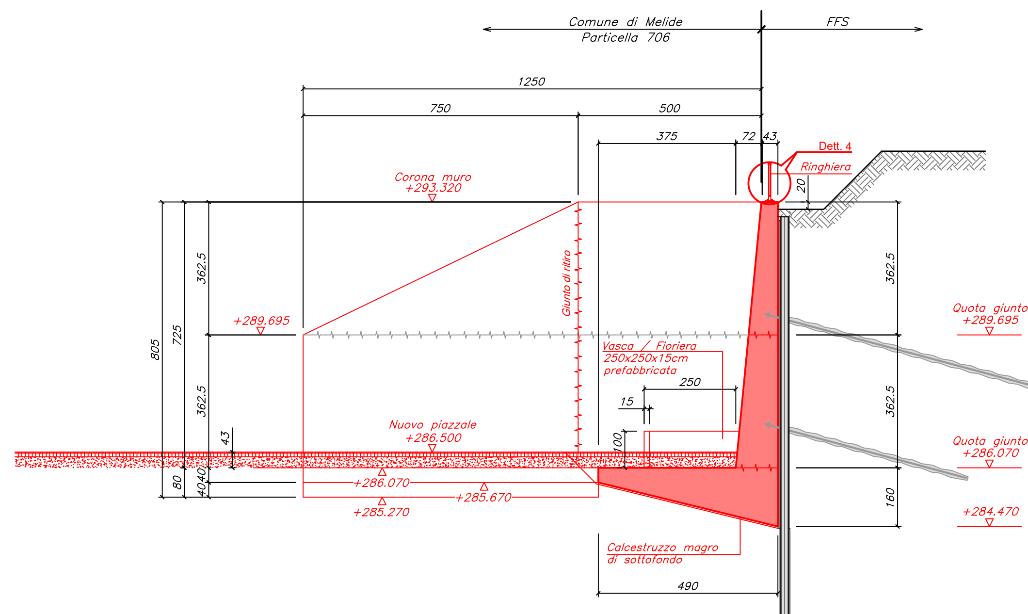
Sezione E-E (1:100)
