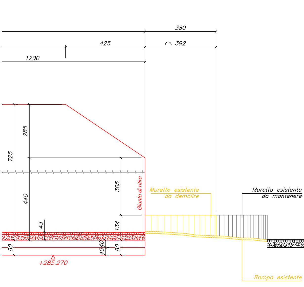
Sezione D-D Demolizione muro (1:100)
