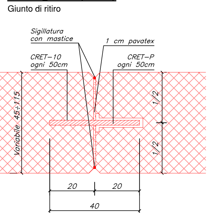
Dettaglio 1 (1:10)
