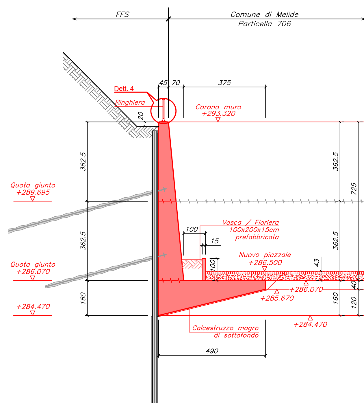
Sezione D-D Demolizione muro (1:100)
