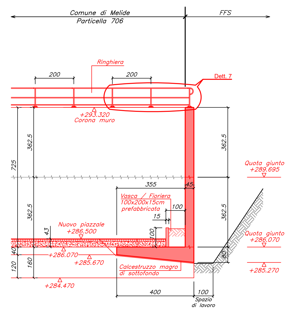
Sezione E-E (1:100)
