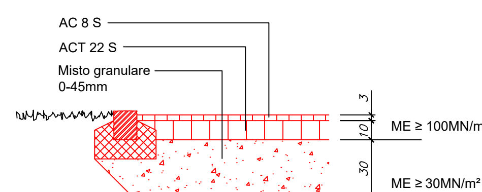
Vista dettaglio 7 (1:20)
