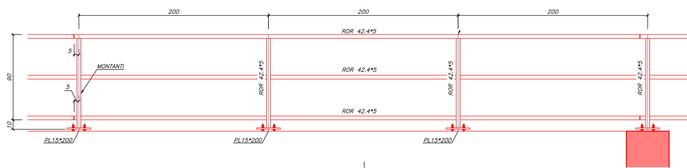
Vista dettaglio 7 (1:20)
