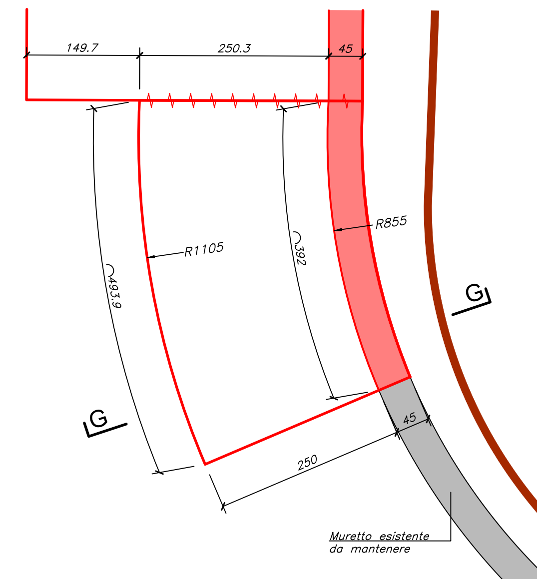
Pianta fondazione muretto in curva (1:50)
