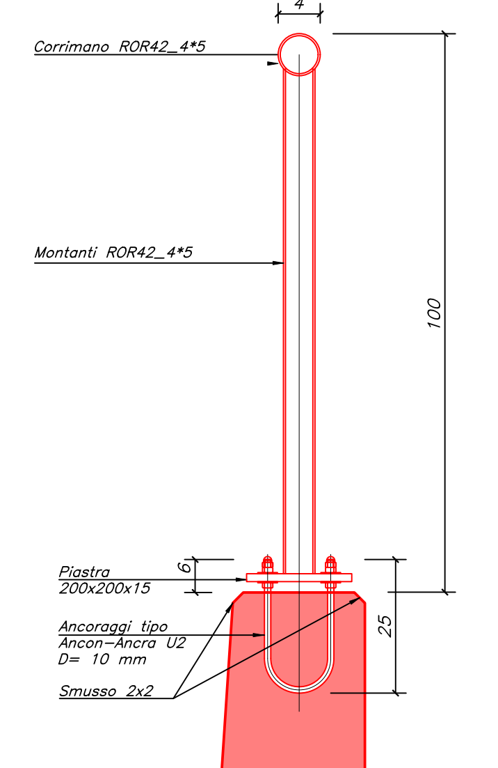
Dettaglio 6 (1:10)
