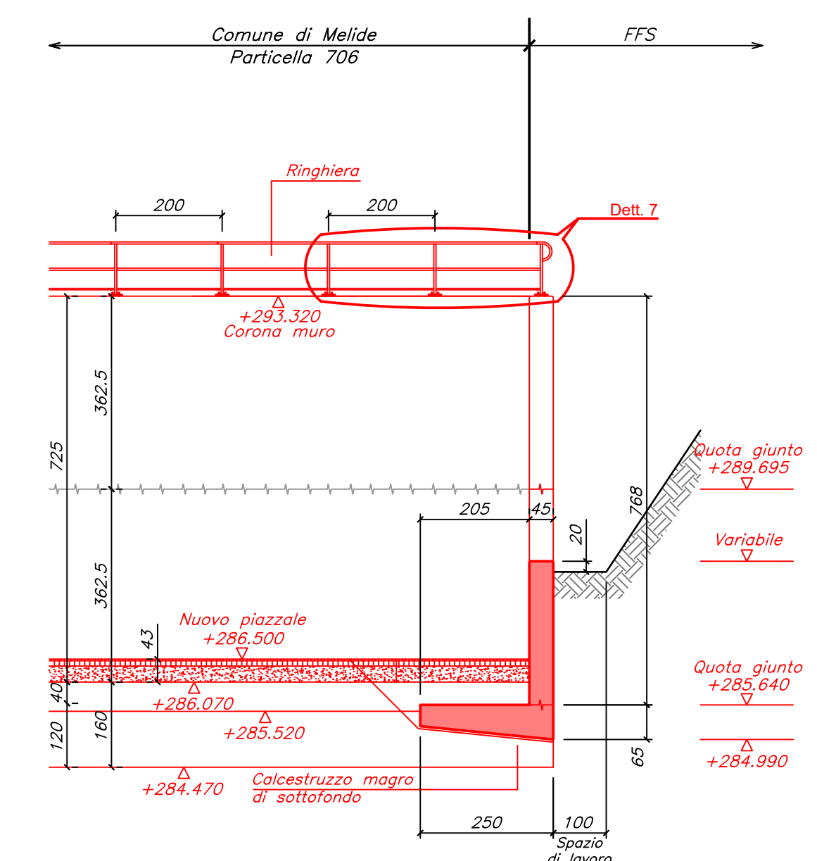
Sezione G-G (1:100)
