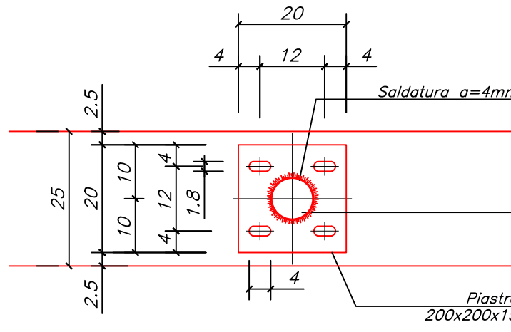
Dettaglio 6 (1:10)
