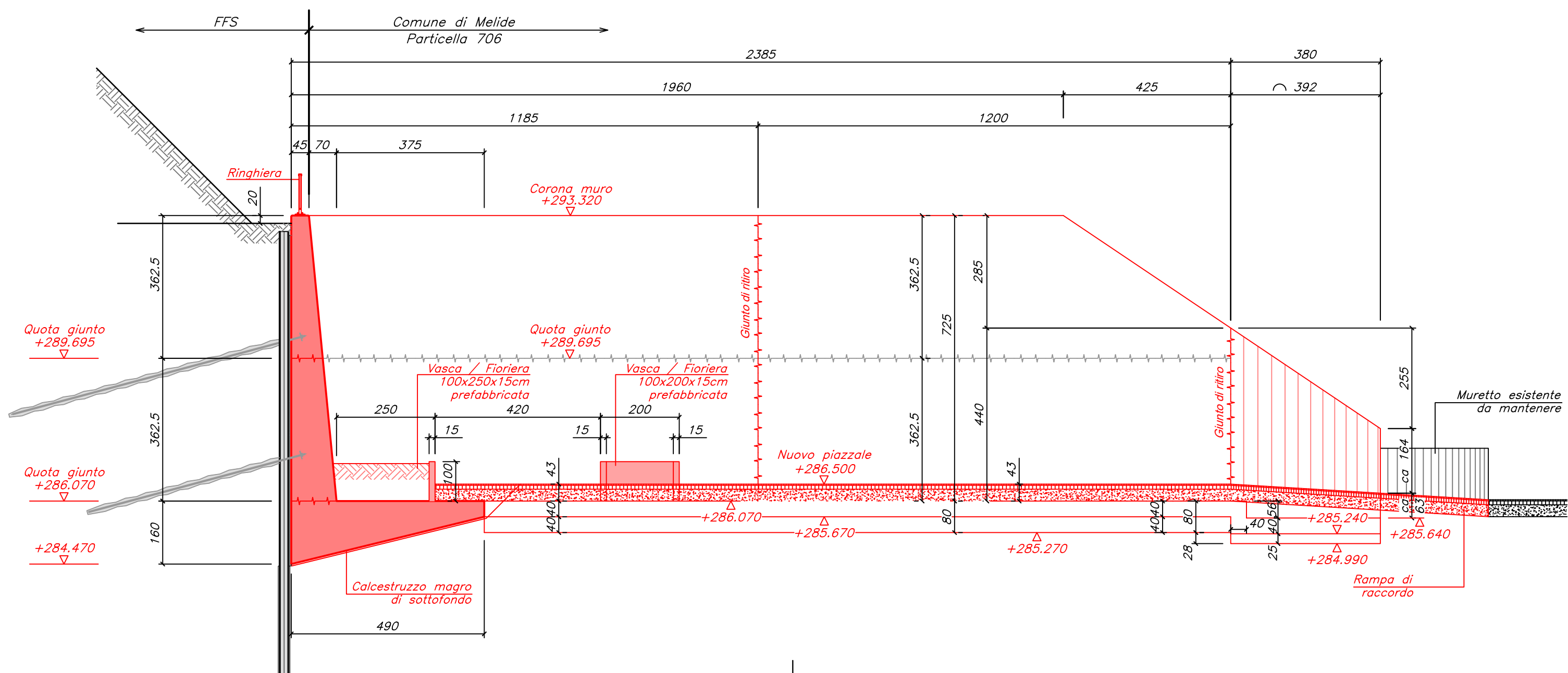
Sezione D-D (1:100)
