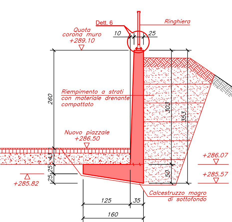
Sezione F-F (1:50)
