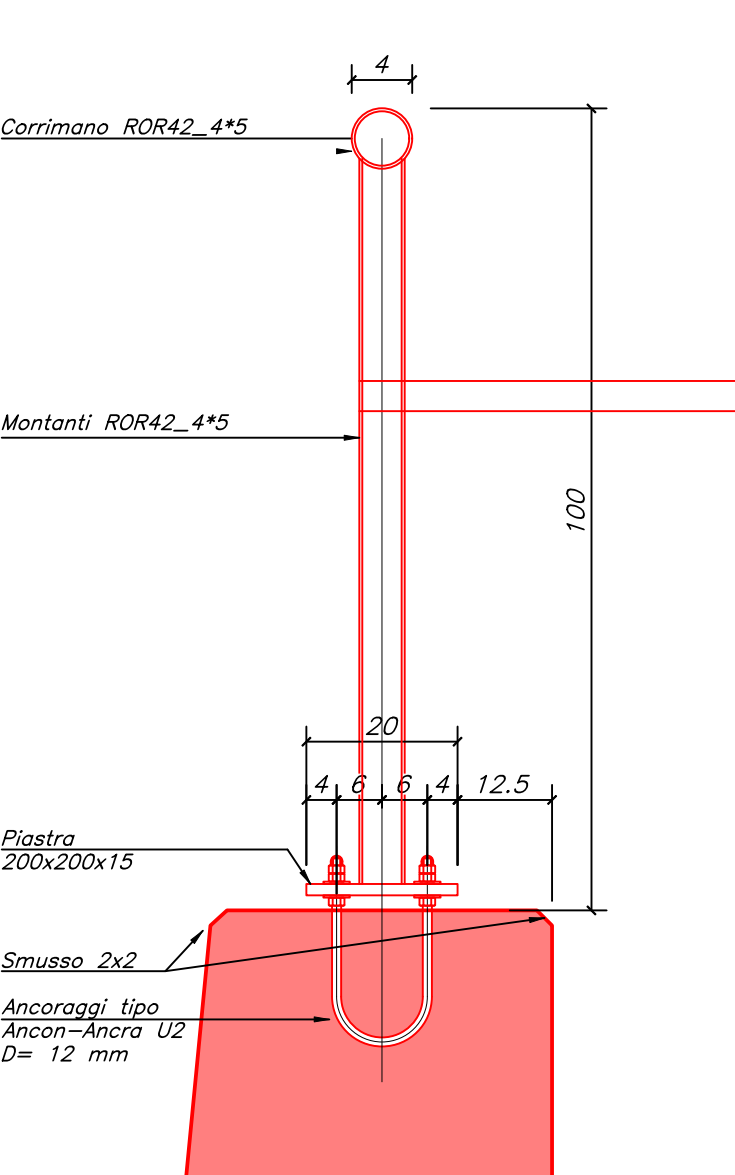
Dettaglio 4 (1:10)
