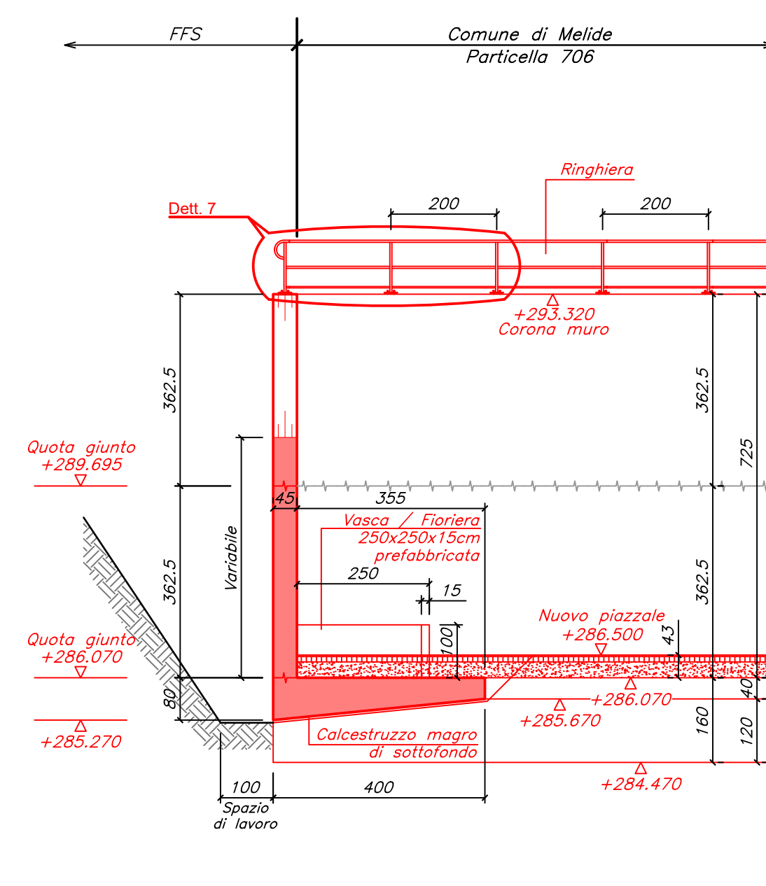
Sezione B-B (1:100)
